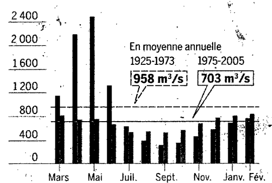
DÉBIT MOYEN ANNUEL DE L'EUPHRATE, 1975-2005, en m 3 /s
